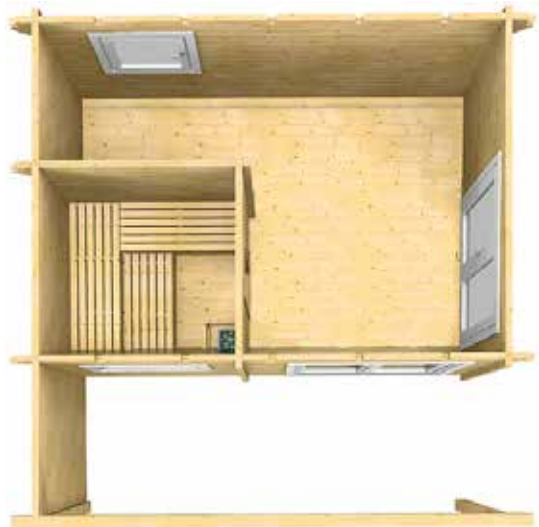
Grundrissbeispiel Blockbohlenbauweise
