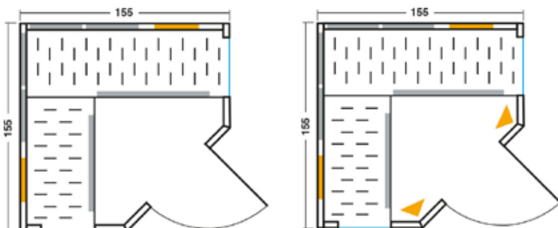
Grundriss Sunlight 155 mit Frontstrahlern
