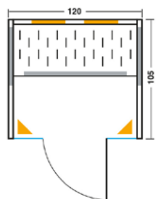
Grundriss Sunlight 120 mit Frontstrahlern
