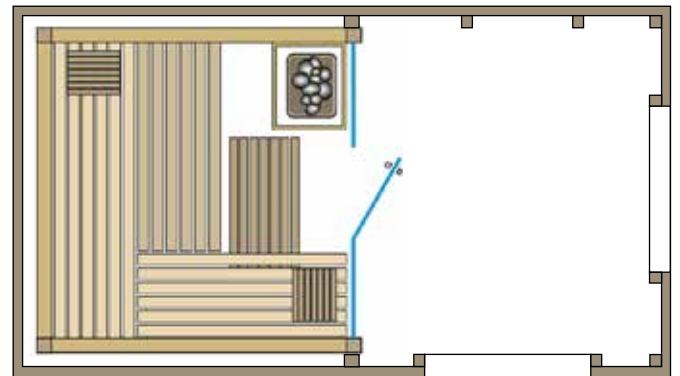
Grundrissbeispiel Elementbauweise
